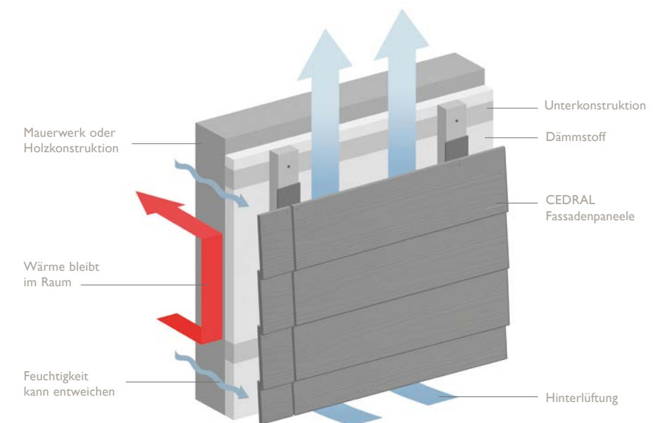
Konstruktionsprinzip der vorgehängten hinterlüfteten Fassade am Beispiel Stülpschalung
